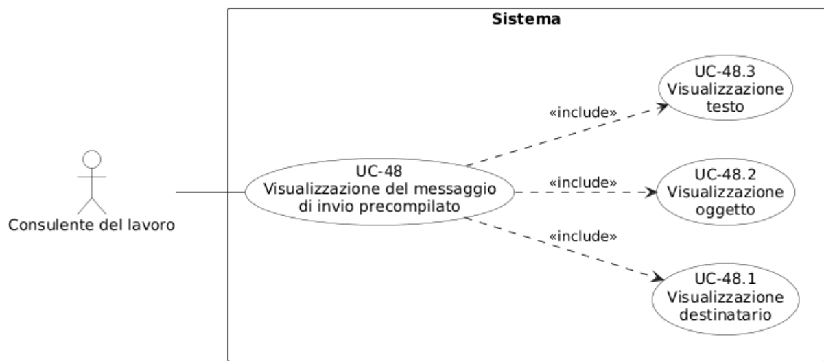
Figura 77: Diagramma del caso d'uso UC-48: Visualizzazione del messaggio di invio precompilato
